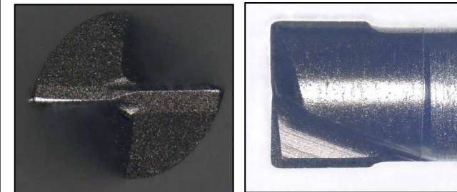
精加工10小时加工后的刀具损伤
