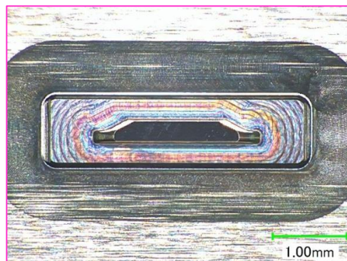
CBN-LRF加工部
